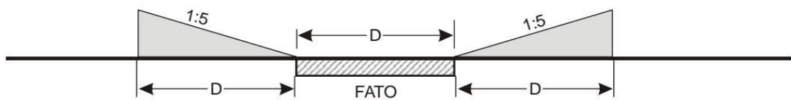
Section A-A
