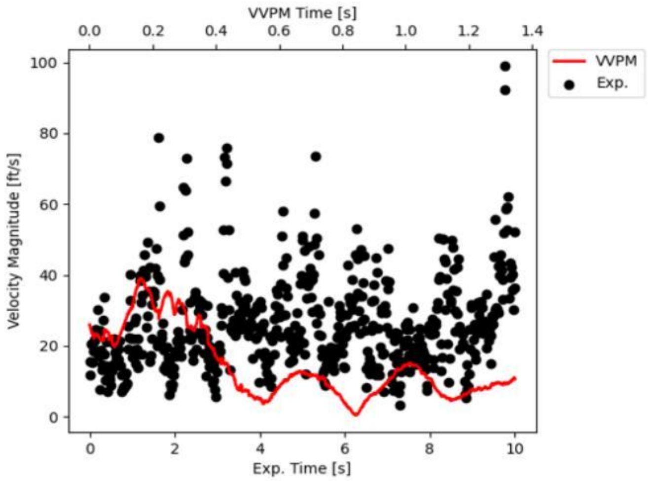
(d) Sensor B2-S10
